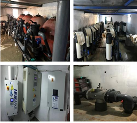
Şekil 9. Su arıtma sistemleri
